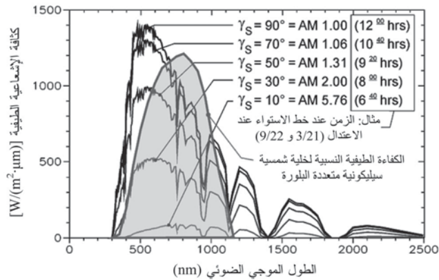
الشكل (2-7): الاستجابة الطيفية الفعلية لخلية شمسية متعددة البلورة (نوع ASE) مع الطيف الشمسي لزوايا ارتفاع مختلفة للشمس، والكتل الهوائية المكافئة (AM)، والزمن عند خط الاستواء للاعتدال.
