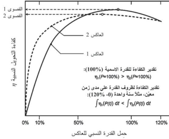
الشكل (28-7): كفاءة التحويل النسبية فقط كدالة في الحِمل النسبي لنوعين مختلفين من العاكسات: فبينما يعطي العاكس 1 كفاءة تحويل قصوى فقط عند الحِمل الاسمي، يعطي العاكس 2 كفاءات عالية لمدى واسع من الأحمال.
