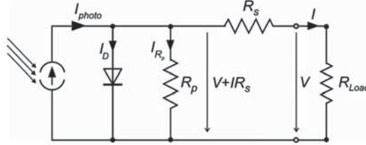
الشكل (12-2): رسم توضيحي للدائرة الكهربائية المكافئة لخلية شمسية وفقاً لـ «نموذج الدايبود الواحد».
