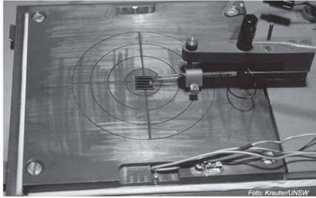
الشكل (2-6): جهاز لقياس خصائص التيار-الجهد ( I-V )، والكفاءة، والاستجابة الطيفية. والشكل مبين مع خلية شمسية ذات كفاءة عالية في جامعة نيو ساوث ويلز (UNSW).
