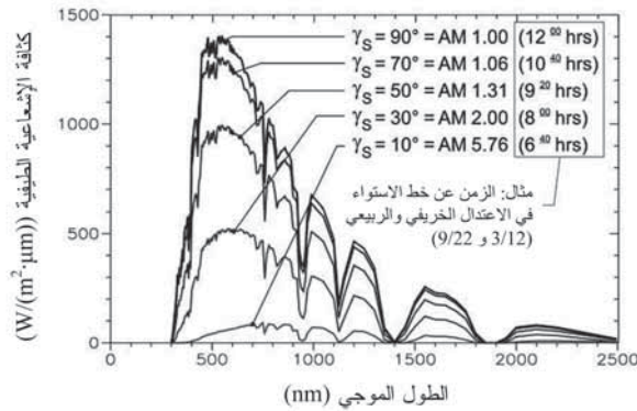
الشكل (7-7): أطيف الإشعاعية الأرضية المباشرة للشمس (AM 1-AM 5.6) وفقاً لنشرة CIE رقم 85 (1990) للكتل الهوائية AM 1، و AM 2، و AM 5.6، وقيم أخرى عن طريق الاستيفاء.
