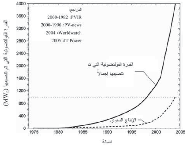
الشكل (21-2): تطور سوق الفولتضوية: السعة التي تم تنصيبها والإنتاج السنوي (المراجع: أخبار الفولتضوية (PV-news) وتقرير المطلعين على الفولتضوية (Photovoltaic Insiders Report (PVIR)- 2000-1982، ومعهد المراقبة العالمية (Worldwatch Institute): 2004، وتقنية معلومات القدرة (IT Power): 2005).
