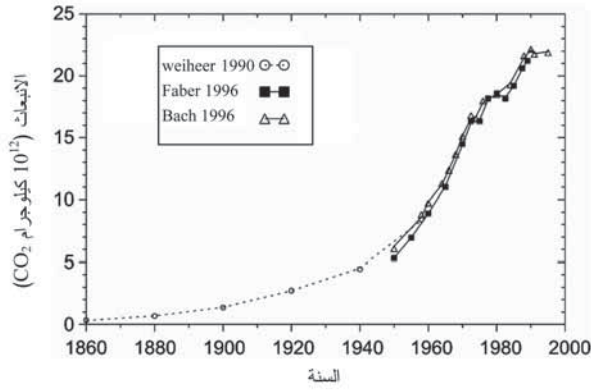
الشكل (3-1): الانبعاثات العالمية البشرية المنشأ لثاني أكسيد الكربون خلال الأعوام (1860-1995) وفقاً لويهير (Weiher) 1990، وفابر (Faber) 1996، وباخ (Bach) 1996، والرصد العالمي (Worldwatch) 2000.
